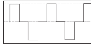
Senoidal modificada de forma de onda producido por el convertidor
