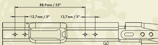
✚ Gewindebohrung/Tapped hole: No. 6-48
