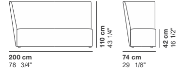
cod. 3516 / B_left element 200 H.110
