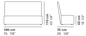
cod. 3507 / B_element 180 H.110
