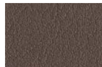
valencia meteor
