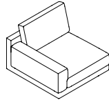
Elle Deep Unit (Left Arm) ELD10L L 104cm D 116cm H 85cm L 41" D 45¾" H 33¾"
