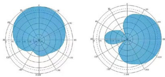
6dBi
