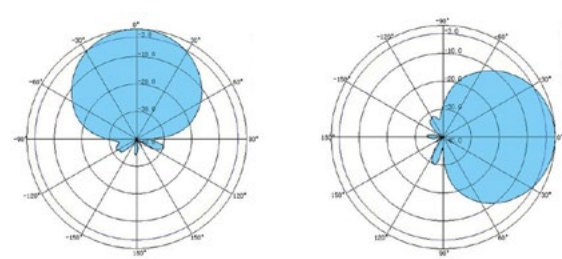
9dBi
