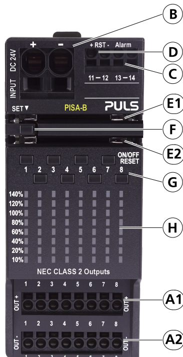
Fig. 13-1: Front side
