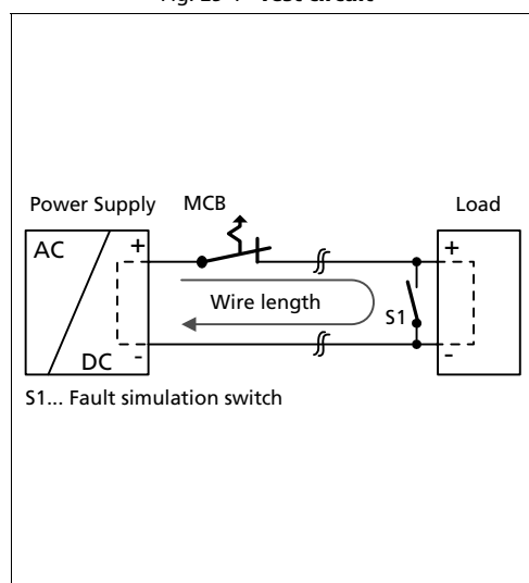
Fig. 25-4 Test circuit
