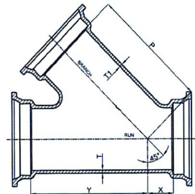
Wyes Lateral 45°
