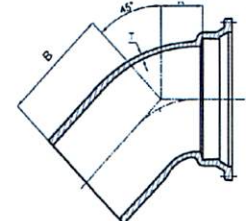
MJ x PE Bend 45°
