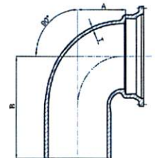
MJ x PE Bend 90°
