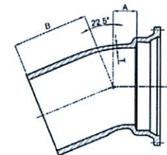
MJ x PE Bend 22-1/2°
