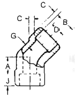
45° ELBOW
