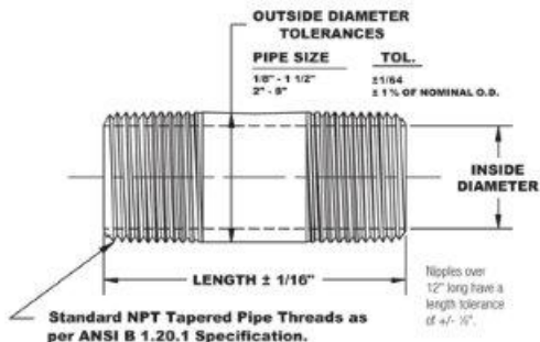
FIG. 343: Standard Galv. Schedule 40
