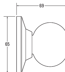
DIMENSIONES (mm)
