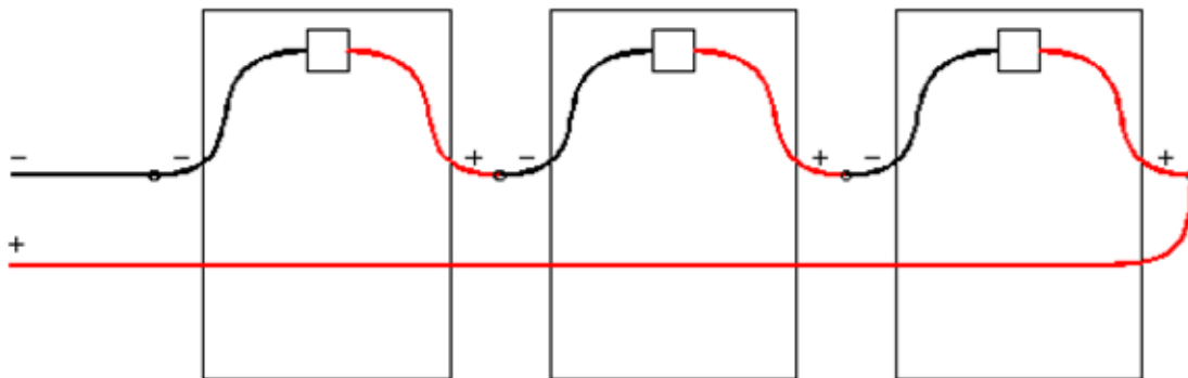
PV Panel Array Wiring
