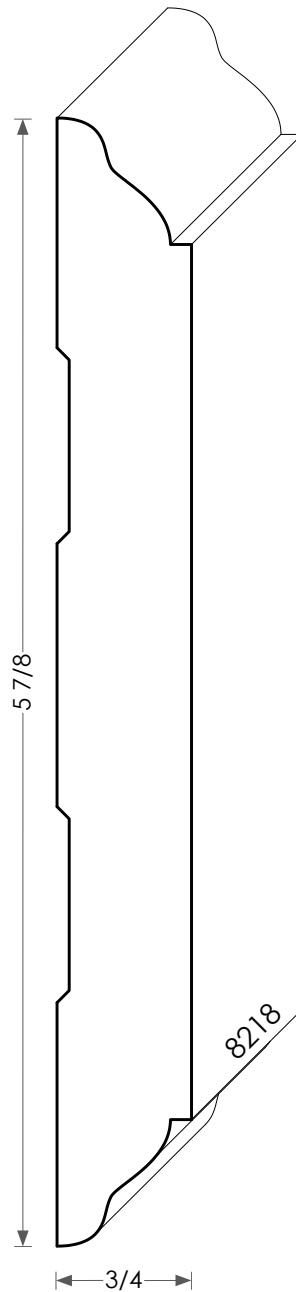
Wood Astragal - 8218
