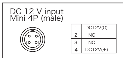
Mini 4P (male) connector
