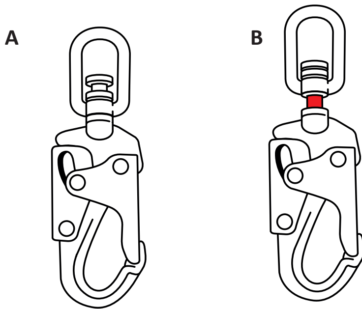
Figura 5: Inspección del Gancho de cierre instantaneo con indicador de carga A Condiciones seguras de funcionamiento normal B Se muestra el indicador visual- Sacar el SRD de Servicio
