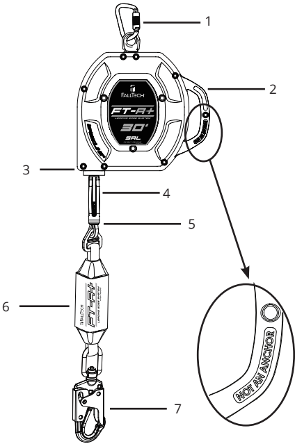
Figure 1 - À propos du bord d'attaque FT-R+ SRL de FallTech® 1 Mousqueton pour la connexion de corde à l'ancrage 2 Poignée de transport (pas une ancre) 3 Ligne de vie du câble 4 Ensemble butée de câble/poignée 5 Oeillet serti 6 Amortisseur d'énergie 7 Mousqueton pivotant en acier
