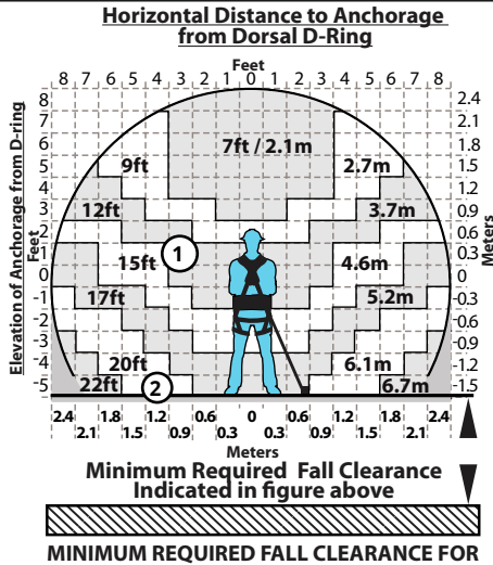
Figure 12 - Dégagement de chute minimum requis pour la FT-X pour les utilisateurs de 59 à 141 kg (130 à 310 lb)
