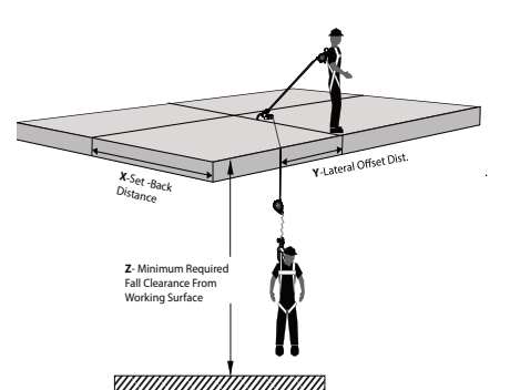
Figure 11 - Ancrage non aérien pour un dégagement minimal requis en cas de chute (DMC)
