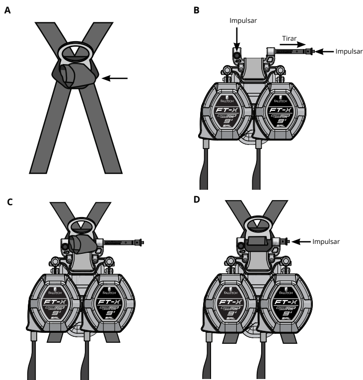
Figura 6 - Instalación de la Cuerda de Salvamento Autorretráctil-P FT-X EdgeCore de Amarre, Arco Eléctrico, Bordes Salientes Clase 2
