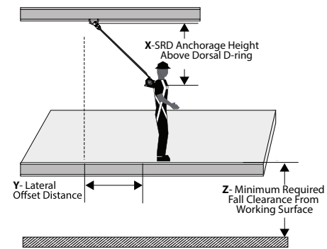
Figure 10 - Ancrage aérien pour dégagement minimal requis en cas de chute (DMC)
