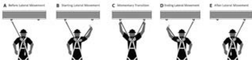
Figura 8 - Cuerda de Salvamento Autorretráctil-P de dos piernas para movimiento lateral
