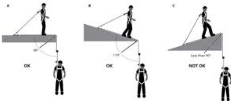
Figure 7 - Angle du bord d'attaque de la redirection de la corde de sécurité
