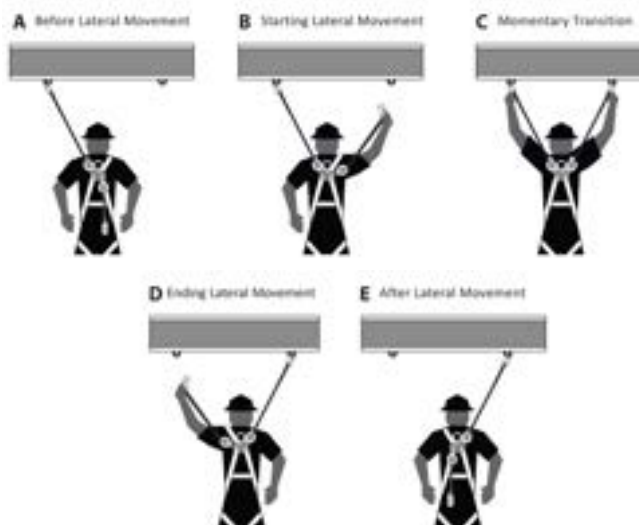
Figure 8 - CSRA-P à deux jambes pour mouvements latéraux
