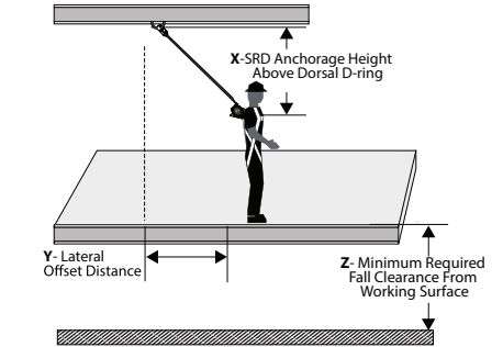
Figure 15 - Le dégagement minimum nécessaire en cas de chute du FT-X pour les utilisateurs de 141 à 191 kg (310 à 420 lb)
