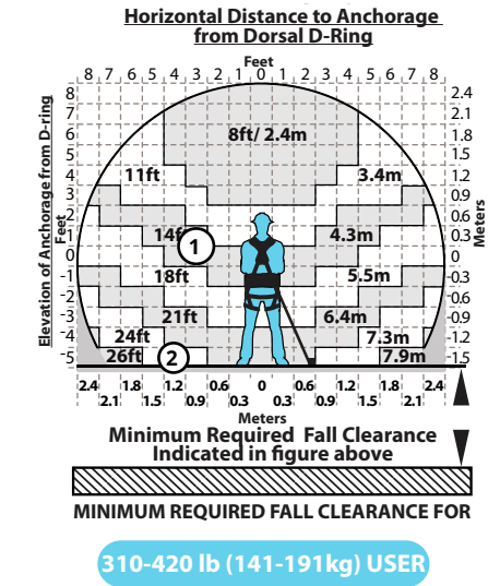
Figure 15 - Le dégagement minimum nécessaire en cas de chute du FT-X pour les utilisateurs de 141 à 191 kg (310 à 420 lb)
