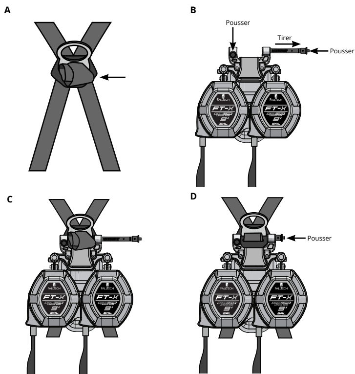
Figure 6 - Installation de la CSRA-P à bord d'attaque de classe 2 avec applications d'arimage à arc électrique FT-X EdgeCore
