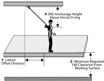
Figure 15 - Le dégagement minimum nécessaire en cas de chute du FT-X pour les utilisateurs de 141 à 191 kg (310 à 420 lb)
