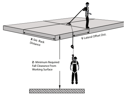
Figure 15 - Le dégagement minimum nécessaire en cas de chute du FT-X pour les utilisateurs de 141 à 191 kg (310 à 420 lb)
