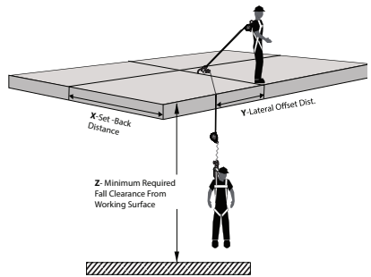
Figura 15: distancia despejada de caída mínima requerida de la FT-X para usuarios de 310 libras a 420 libras (141 kg a 191 kg)
