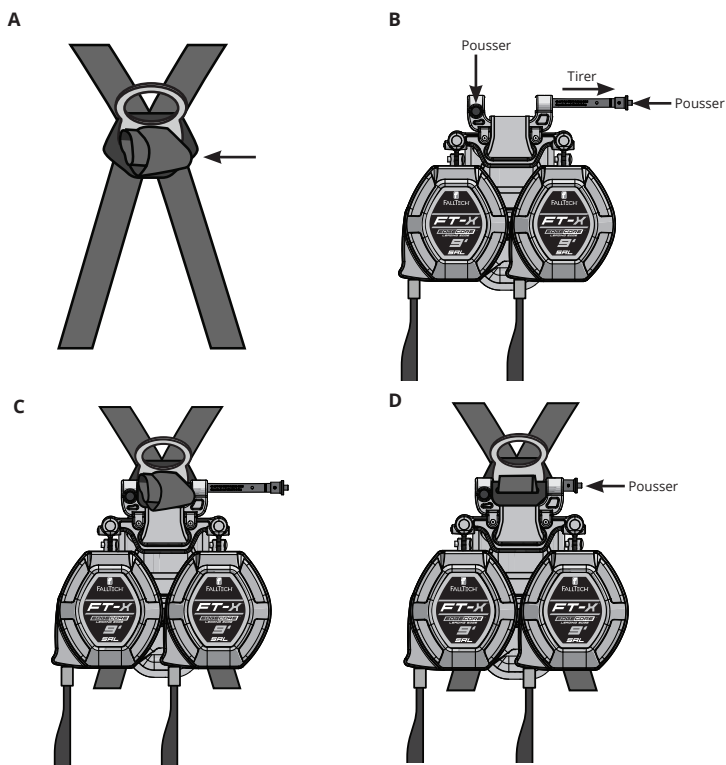
Figure 6 - Installation de la CSRA-P à bord d'attaque de classe 2 avec applications d'arrimage à arc électrique FT-XTM EdgeCore™
