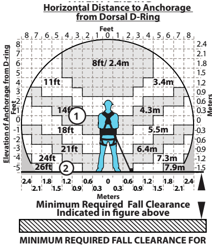
Figura 15: distancia despejada de caída mínima requerida de la FT-X para usuarios de 310 libras a 420 libras (141 kg a 191 kg)
