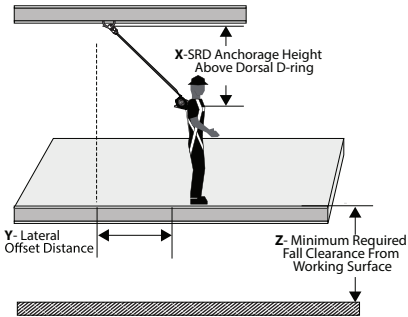
Figura 15: distancia despejada de caída mínima requerida de la FT-X para usuarios de 310 libras a 420 libras (141 kg a 191 kg)
