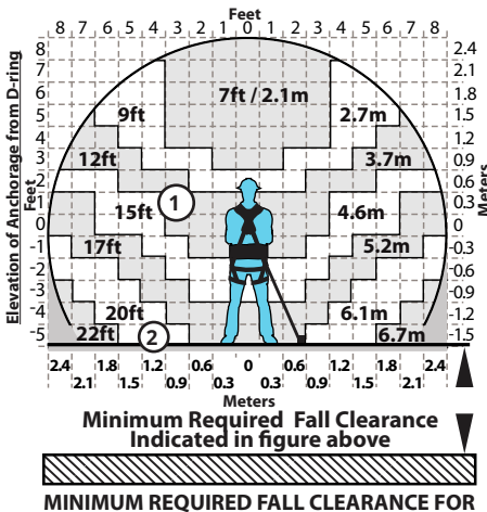
Figura 12 - Distancia despejada de caída mínima requerida de FT-X para usuarios de 130 a 310 libras (59 a 141 kg)
