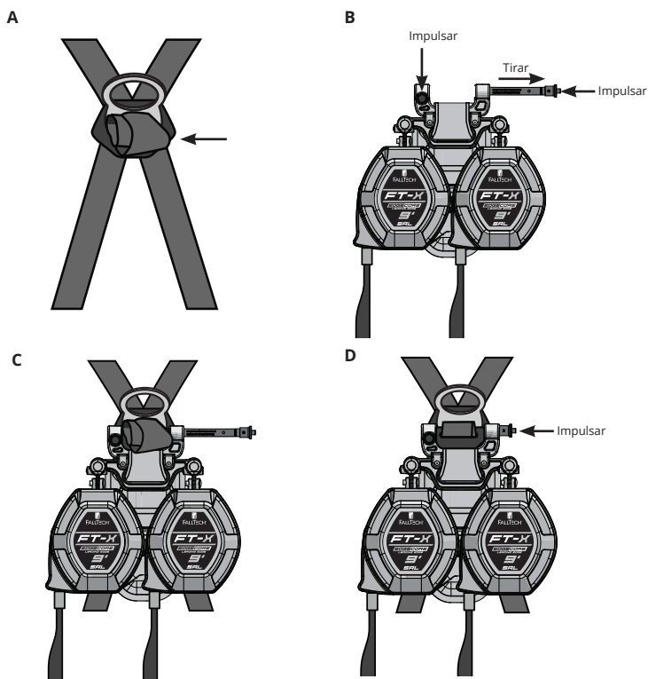
Figura 6 - Instalación de la Cuerda de Salvamento Autorretráctil-P FT-XTM EdgeCore™ de Amarre, Arco Eléctrico, Bordes Salientes Clase 2
