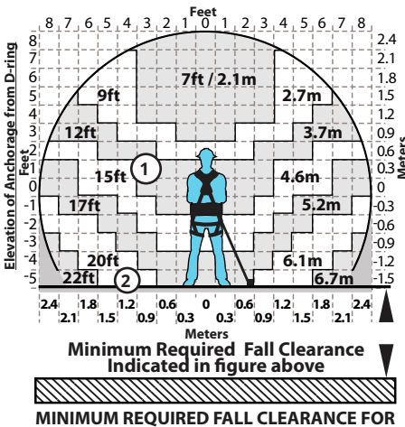
Figure 12 - Dégagement de chute minimum requis pour la FT-X pour les utilisateurs de 59 à 141 kg (130 à 310 lb)
