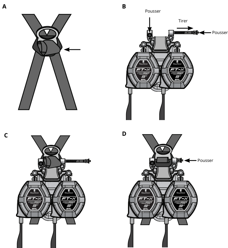
Figure 5 - Installation de la CSRA-P à bord d'attaque FT-X EdgeCore à arc électrique de classe 2
