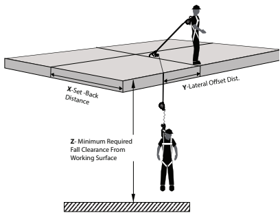
Figura 13 - MRFC en anclaje no suspendido
