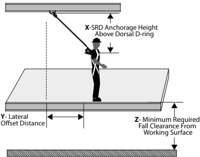
Figura 12 - Anclaje suspendido de MRFC
