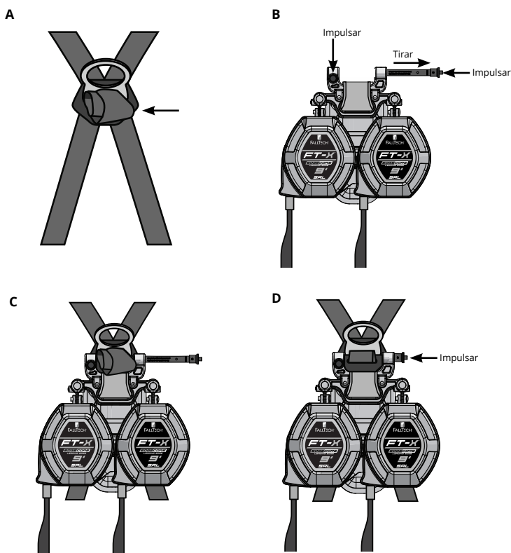
Figura 5 - Instalación de la Cuerda de Salvamento Autorretráctil-P FT-X EdgeCore™, Arco Eléctrico, Bordes Salientes Clase 2
