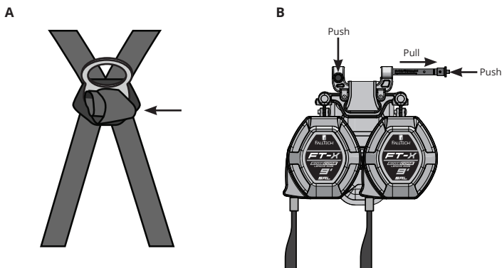
Figura 5 - Instalación de FT-X Cable Class 2 Leading Edge SRL-P
