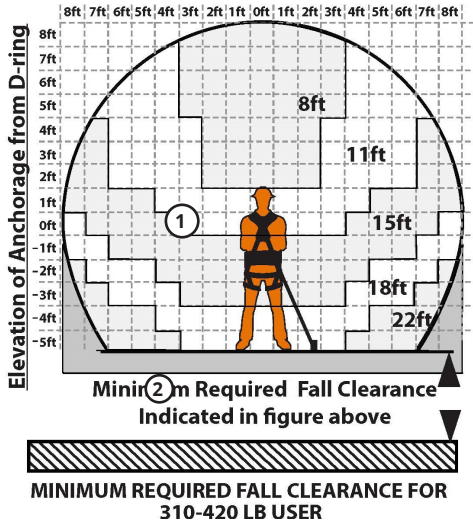
Figure 14 - Dégagement de chute minimum requis pour le FT-X pour les utilisateurs de 141 à 191 kg (310 à 420 lb)
