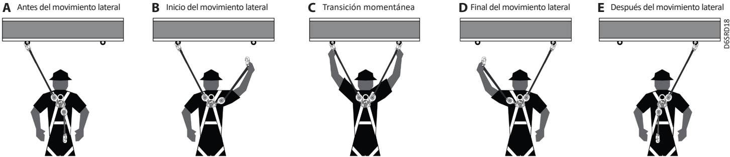
Fig.8: Uso del SRD doble para el movimiento lateral A Ubicación de trabajo original antes del movimiento lateral B A partir del movimiento lateral; una pierna conectada al anclaje C Durante el movimiento lateral; ambas piernas conectadas en transición momentánea entre los anclajes D Final del movimiento lateral; una pierna conectada al anclaje E Nueva ubicación de trabajo después del movimiento lateral T6SRD18
