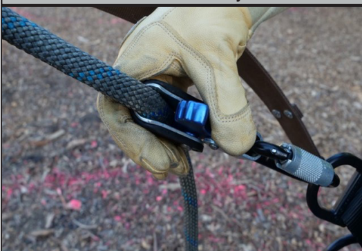
Illustration 15 : Libération de l'ajusteur de corde
