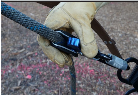
Figura 15: Liberación del ajustador de cuerda
