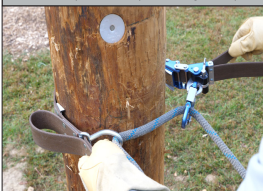
Illustration 7A : Déplacement de l'ajusteur de sangle vers le poteau
