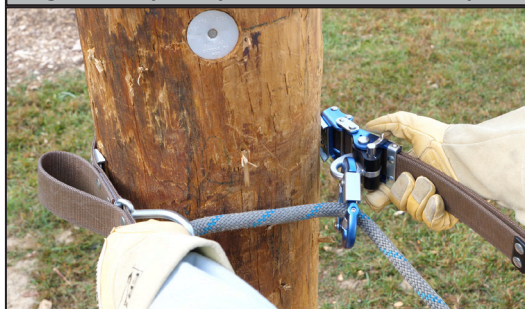
Figura 8: Alejar el ajustador de la correa del poste
