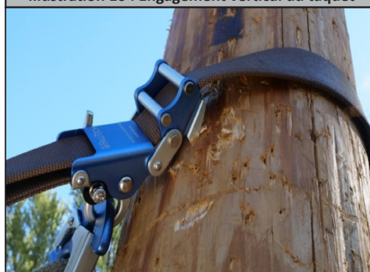
Illustration 10 : Engagement vertical du taquet
