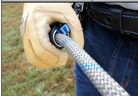
Illustration 16 : Libération de l'ajusteur de câble
