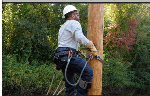
Illustration 19 : Hauteur de la sangle pour le repositionnement
