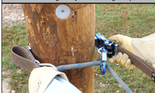
Illustration 8 : éloigner l'ajusteur de sangle du poteau
